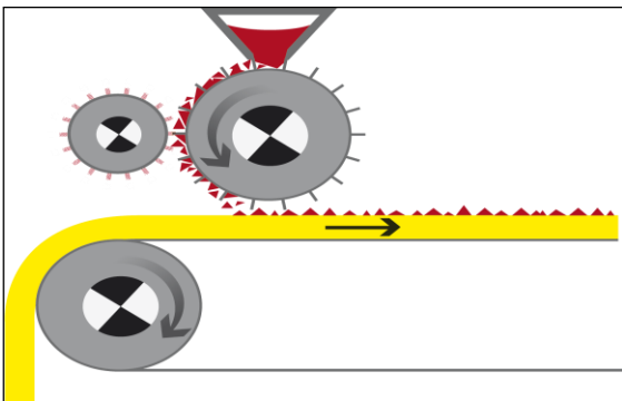
(Funktionsprinzip der Pulverstreubeschichtung)
